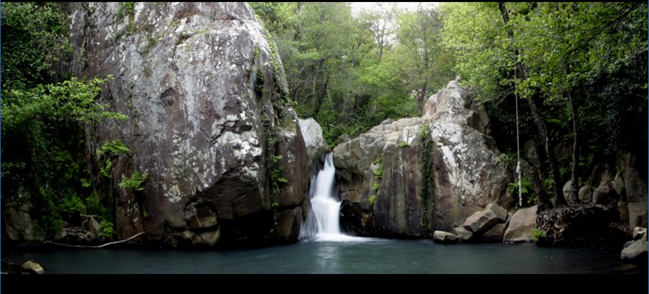
Cascada Río de La Miel. Areniscas del Aljibe, Burdigaliense, Terciario. Algeciras. SE de Sierra de Luna, NW Hoja de La Línea. (por Juanlu Gonzalez-Google)
