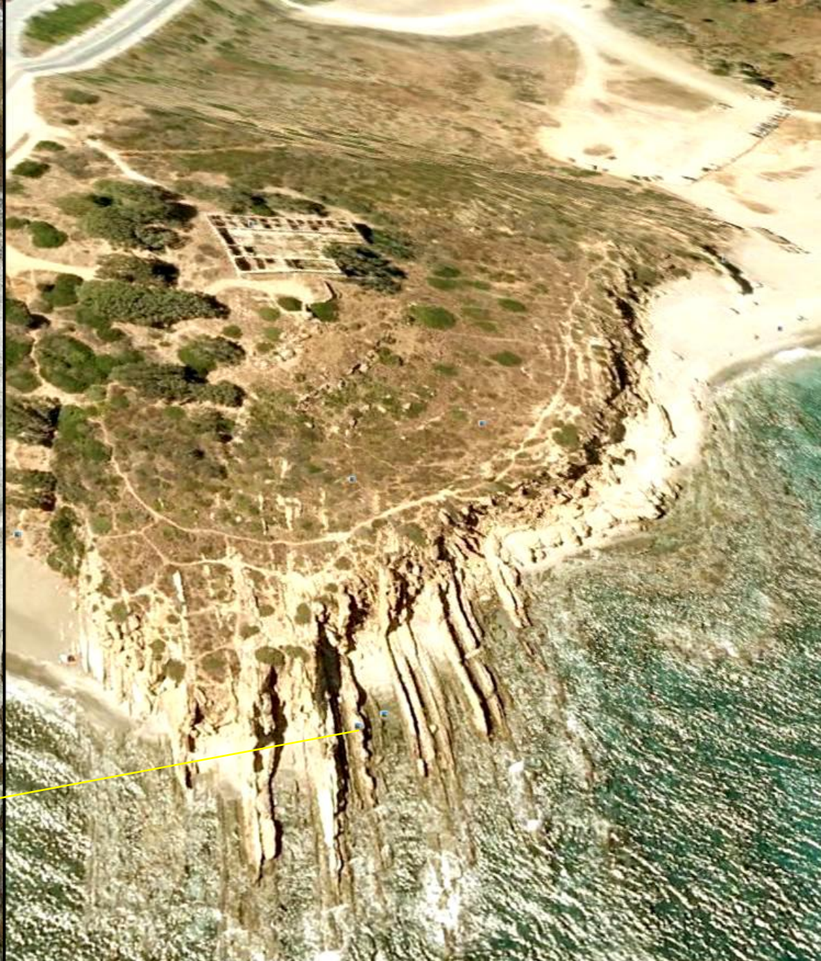
Entrada en el mar de los estratos verticales del Terciario al N de Torreguadiaro
