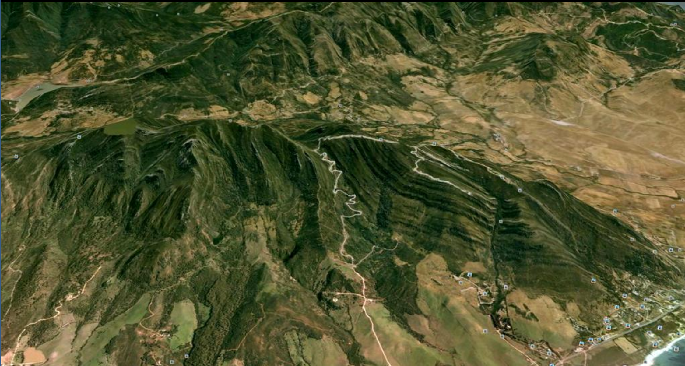
Perspectiva desde el NW – relieve realzado- de la Sierra de Enmedio. Con Areniscas del Aljibe, Burdigaliense, Terciario. Fuerte tectónica. SW Hoja de Tarifa.
